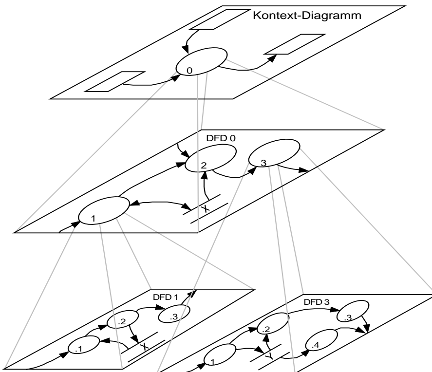
BILD 7.20. Beispiel einer DFD-Hierarchie in Strukturierter Analyse
