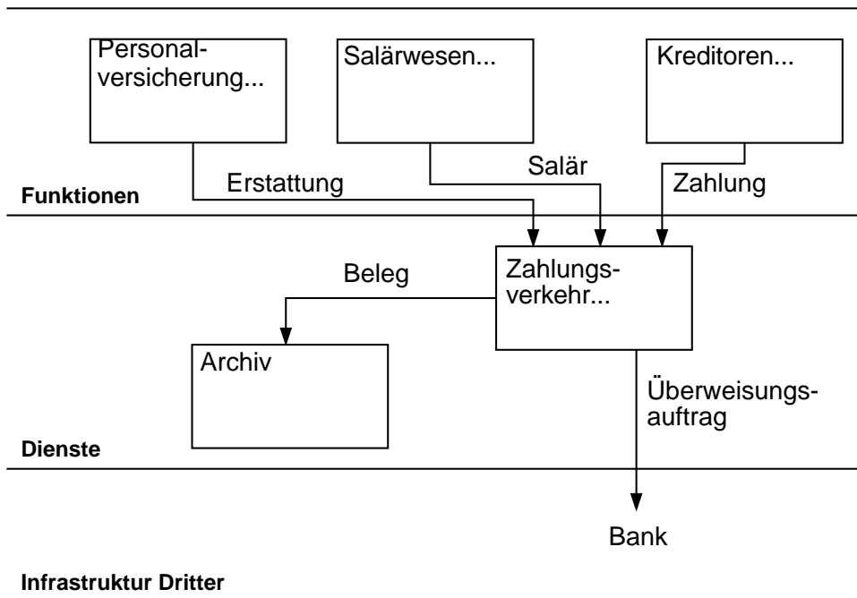
BILD 7.16 b. ... durch Delegieren von Aufgaben und Anordnung der Aufgaben in Schichten übersichtlich und anschaulich modellieren
