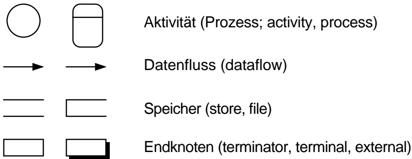
BILD 7.19. Notationen für Datenflussdiagramme
