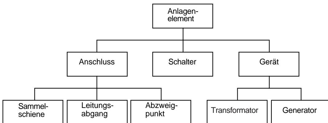
BILD 7.17. Generalisierungsabstraktion – Problemgerechte Modellierung der Begriffswelt der Realität am Beispiel des Engineerings von Unterstationen in Stromverteilungsnetzen
