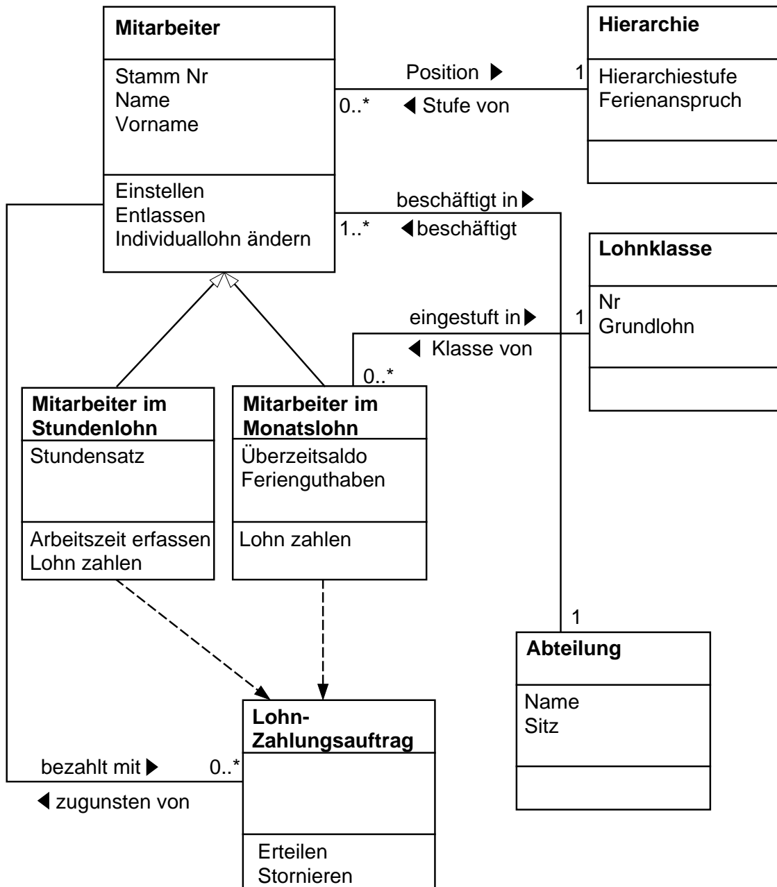
BILD 7.22. Beispiel eines Klassenmodells (stark vereinfachtes Modell eines Personalinformationssystems)
