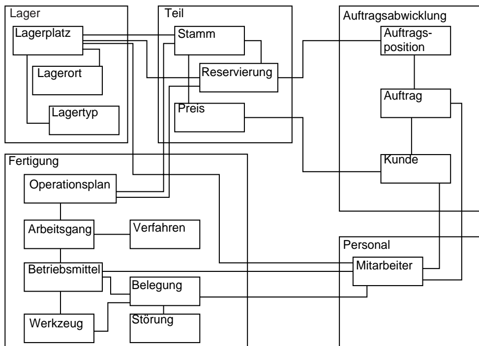
BILD 7.15 b. ...durch Bildung übergeordneter Komponenten...
