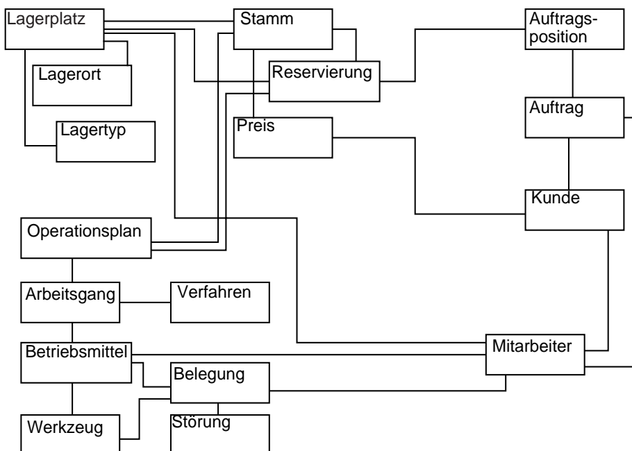
BILD 7.15 a. Kompositionsabstraktion – Komplexe Gebilde mit vielen Komponenten...
