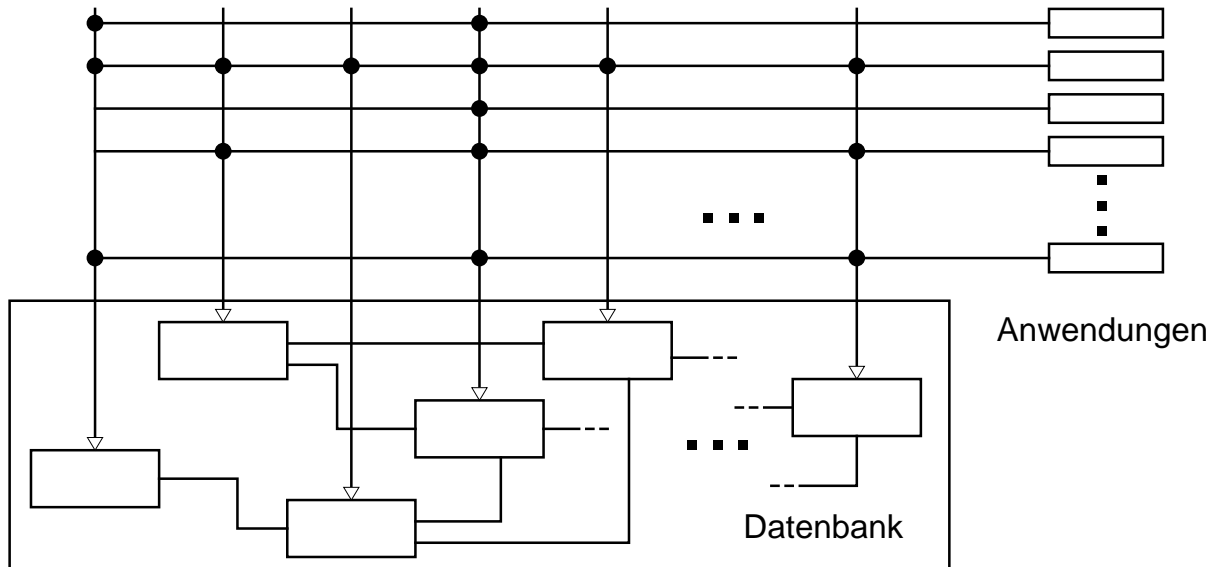
BILD 6.8. Architektur eines datenbankbasierten Anwendungssystems nach dem Matrixmuster
