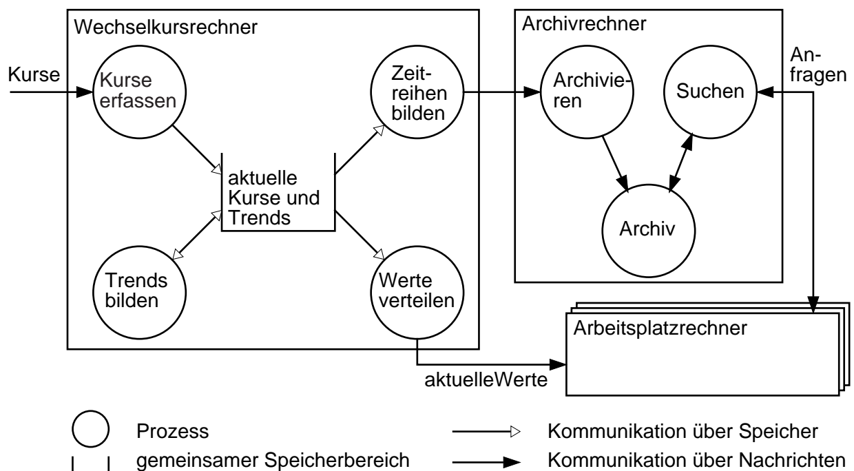
BILD 6.5. Beispiel einer prozessorientierten Architektur
