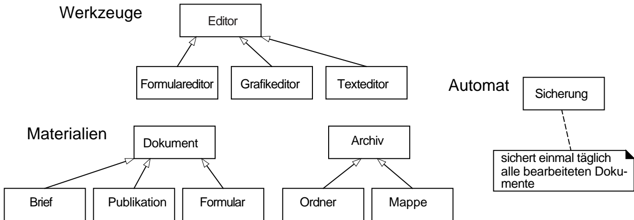
BILD 6.9. Die WAM (Werkzeug-Automat-Material)-Metapher
