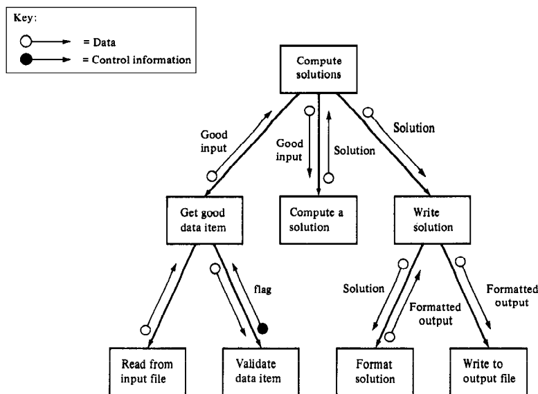
BILD 6.2. Funktionsorientiert gegliedertes System
