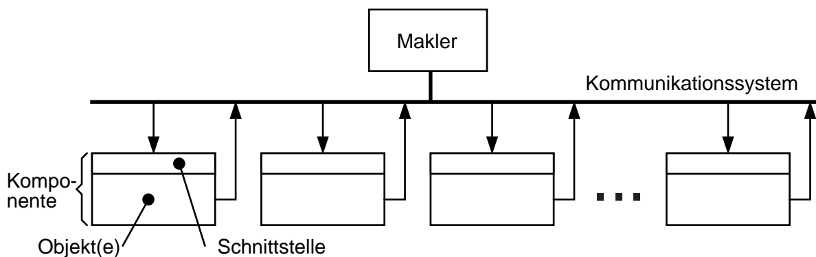
BILD 6.6. Beispiel einer komponentenorientierten Architektur
