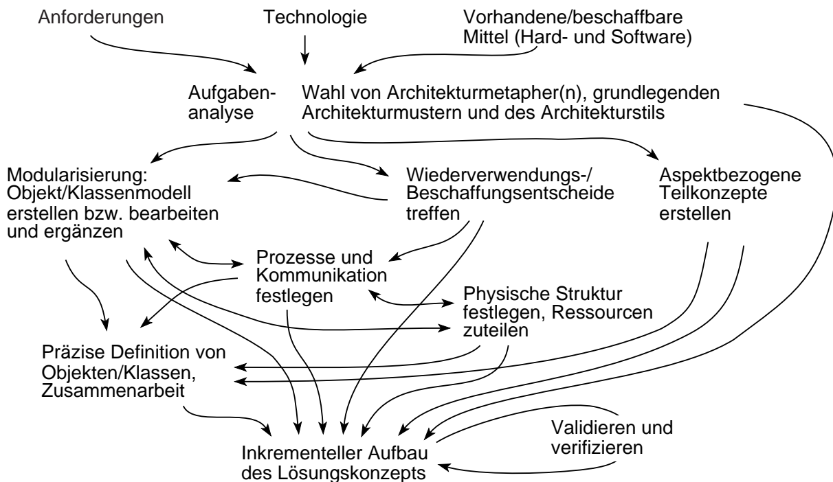
BILD 6.1. Zusammenhänge zwischen den Aufgaben des Architekturstils (am Beispiel eines objekt-orientierten Entwurfs)
