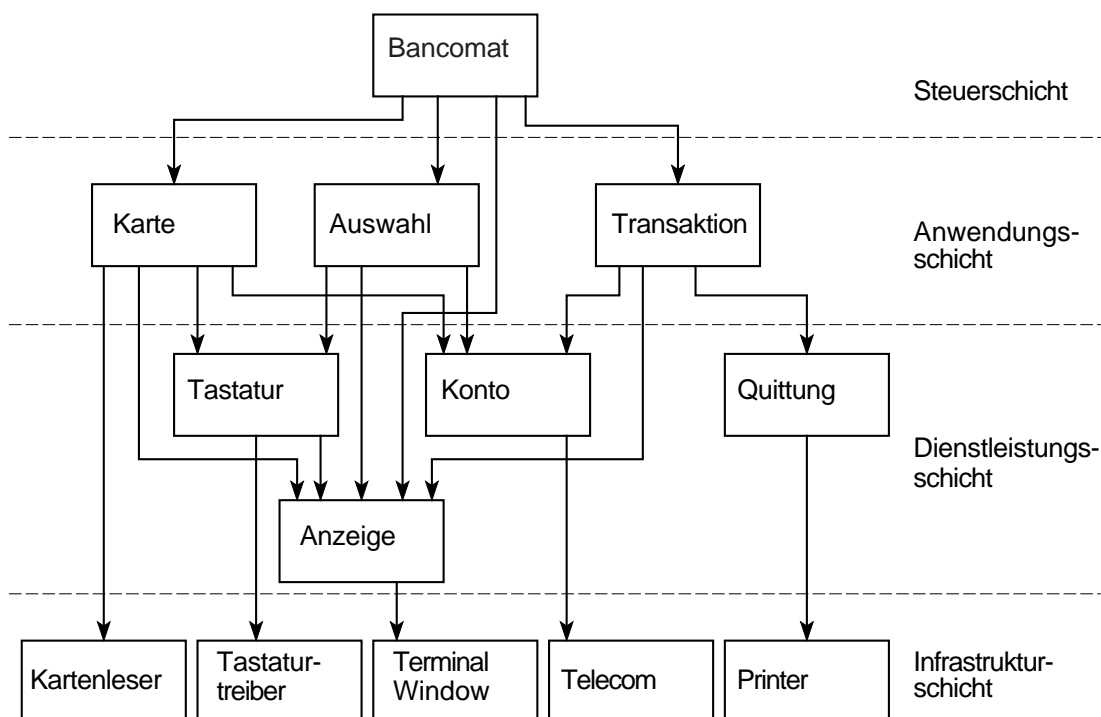
BILD 6.3. Benutzungshierarchie und Schichtung im Entwurf mit Datenabstraktionen
