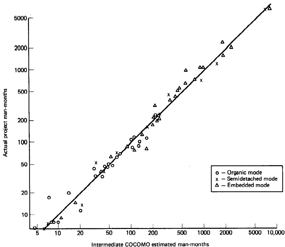
BILD 5.3. Genauigkeit von COCOMO-Schätzungen
