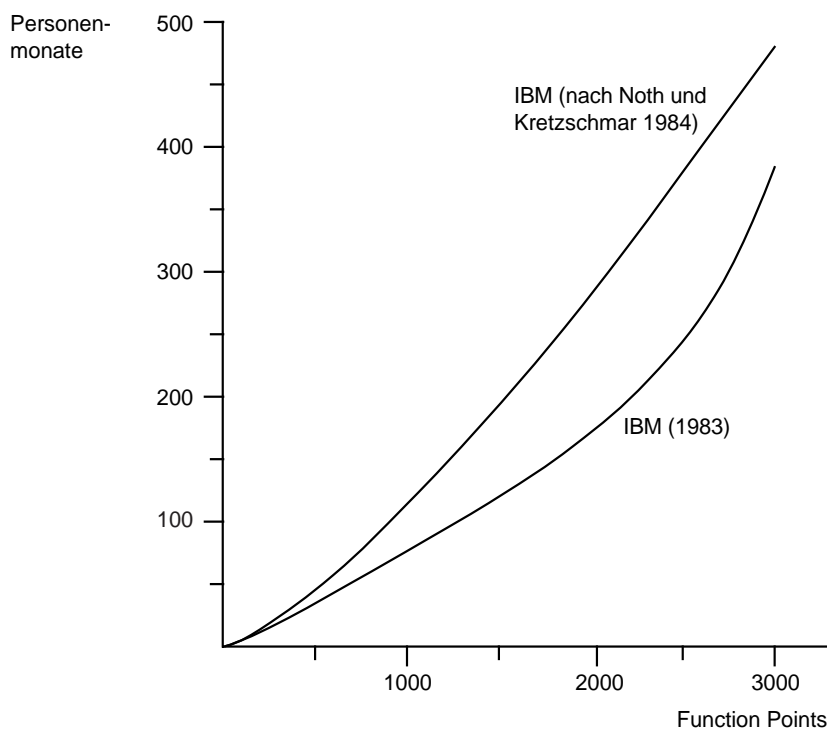
BILD 5.6. Bestimmung des Aufwands aus den Function Points
