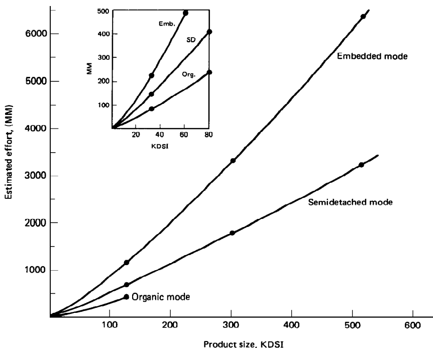
BILD 5.4. Aufwandsschätzung nach COCOMO
