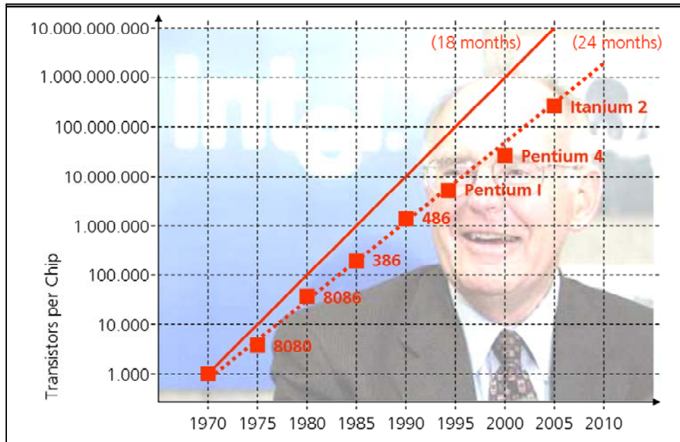
Abbildung 25: Moore'sche Gesetz
