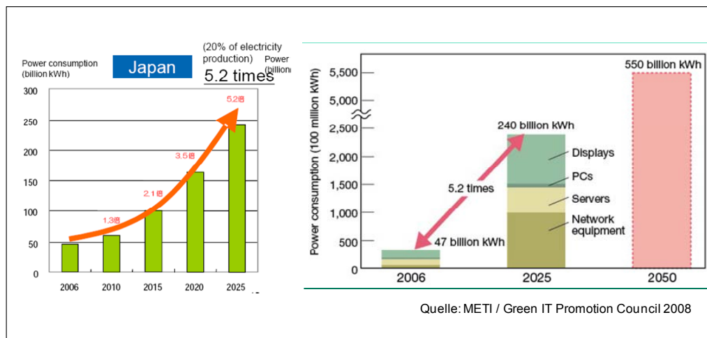
Abbildung 44: METI Prognose des IKT-Stromverbrauchs in Japan [METI 2008]
